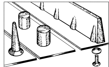
Påskruvade medbringare
